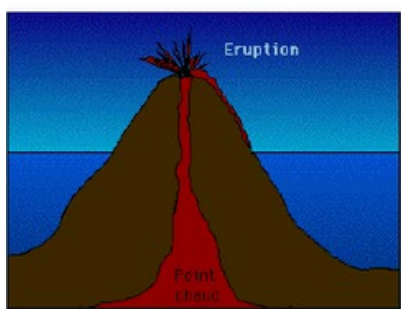
Formation du volcan par accumulations de matériel basaltique.
