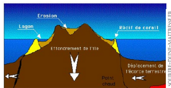
Fin du volcanisme, érosion et transformation de l'île.
