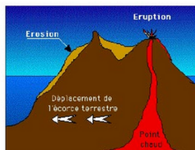
Déplacement de la plaque et formation d'un 2 ème volcan.
